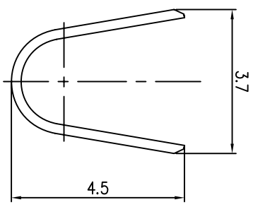
SEC A-A'
